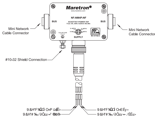
FIGURE 4. Mini Powertap
