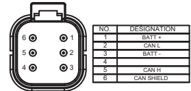
DEUTSCH PLUG DETAIL
